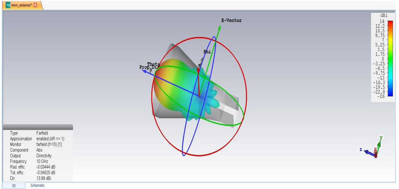
Şekil 1. Horn antenin 3 boyutlu uzak-alan ışınma örüntüsü.
